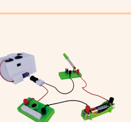
理化實驗-數控電流磁效應
